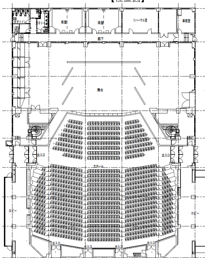
【大ホール】
