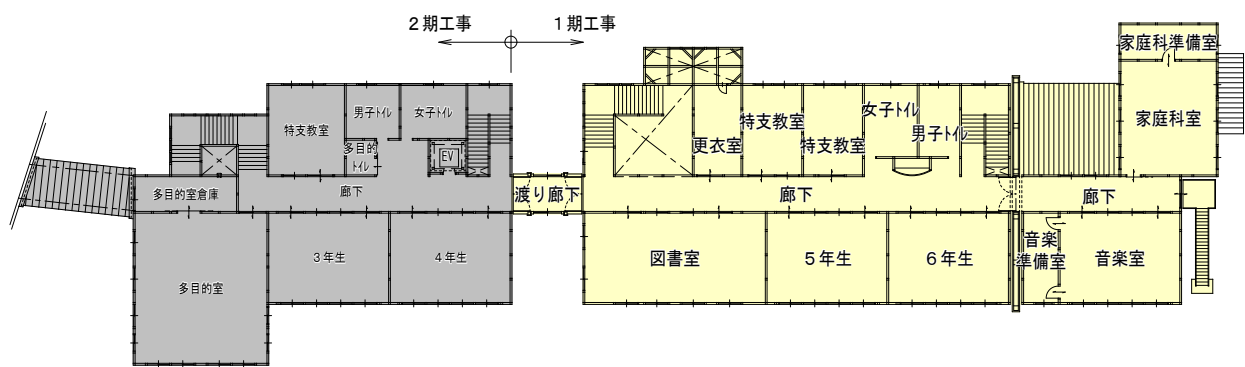
2 階 平 面 図
