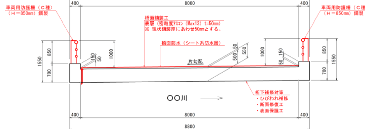
補修図（一般図）
